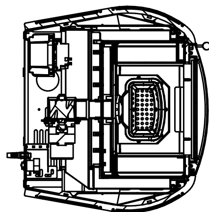
SEZ. A-A
